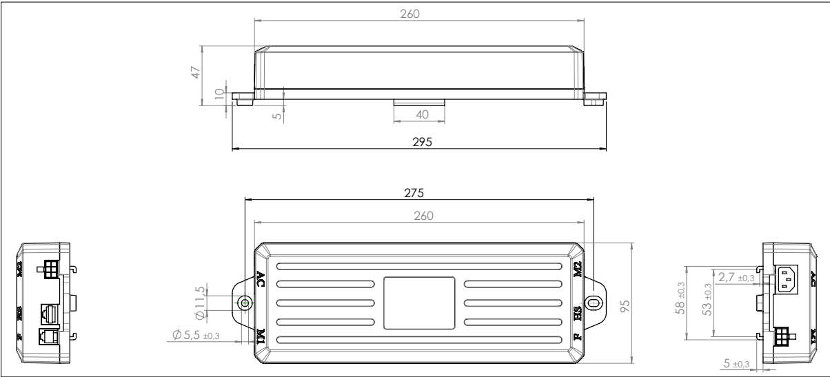
Befestigungsmaße des Steuergerätes für Tischsäule 1 E / 2 E
