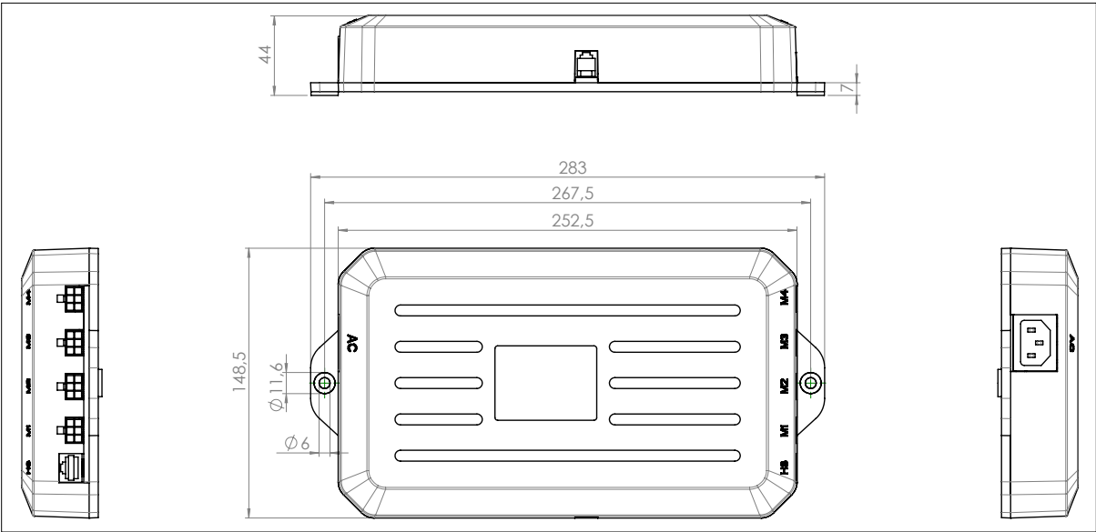
Befestigungsmaße des Steuergerätes für Tischsäule 3 E / 4 E / 6 E / 8 E
