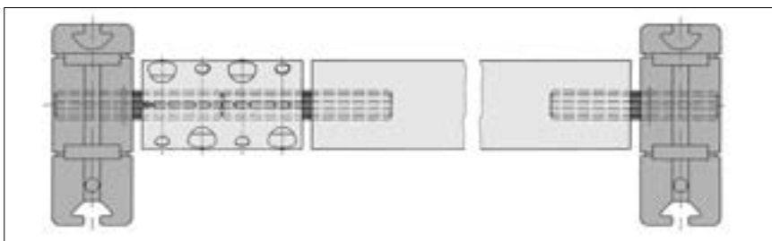
Verbindung von Zahnriemenumlenkungen mit Abständen von mehr als 500 mm mit Synchronwelle.
